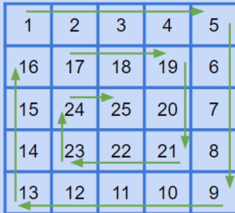
Ma trận xoáy ốc cỡ 5x5
